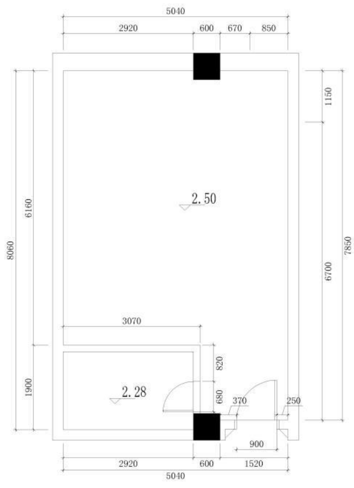
天花标高图 1:50
